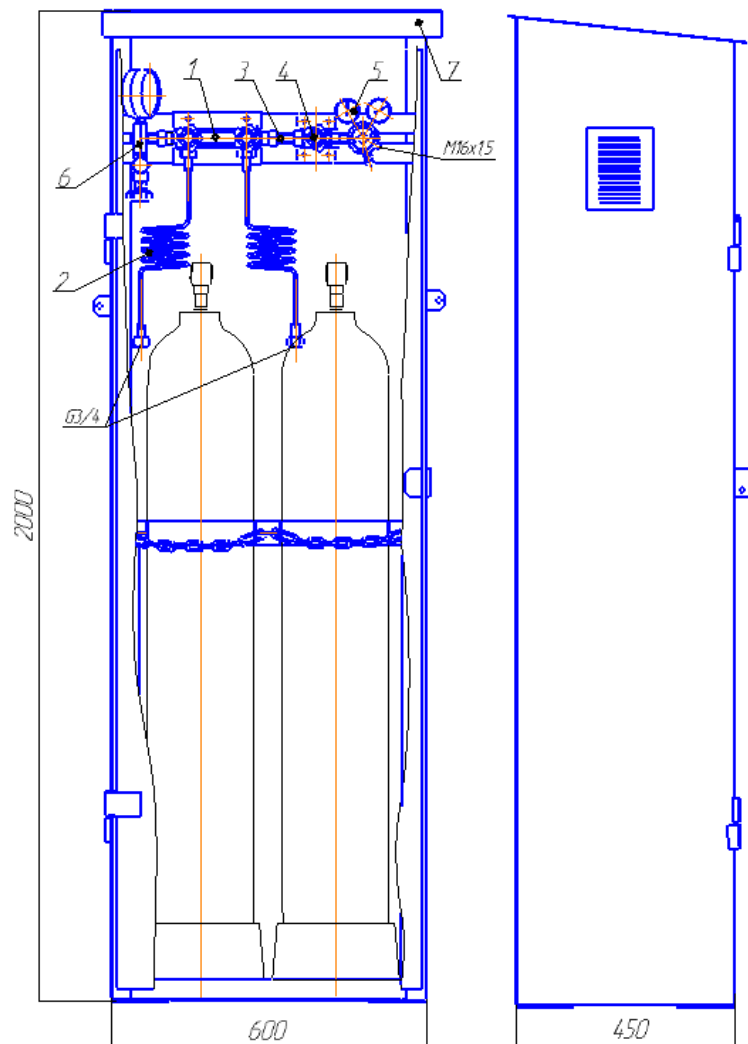
Схема рампы разрядной РР-01(2ш 1х2)
