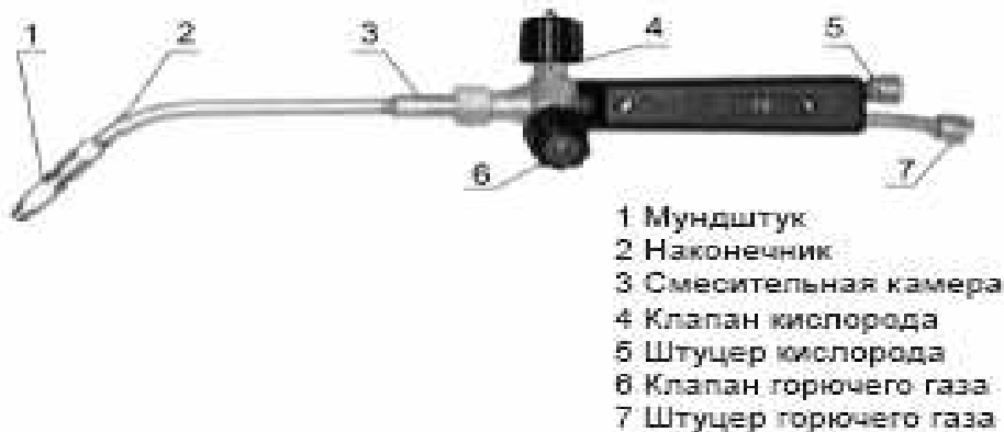
Рис.1 Горелка Г-3, Г-3У
